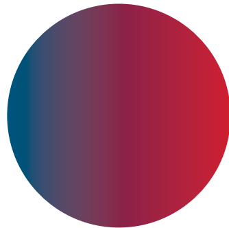
STURM GRADIENT
