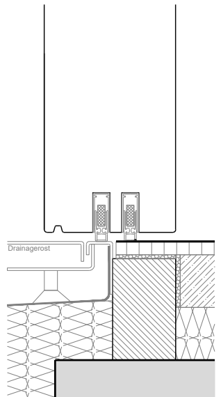
Streiftür mit Drainagerost (nicht geeignet für stark bewitterte Bereiche)
