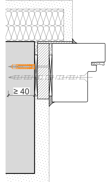
Leibungsmontage mit Blindstock
