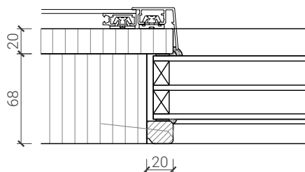
Glas mittig, 68 mm Glasleiste einseitig und Aluminium Vorsatzschale aufgekleipt
