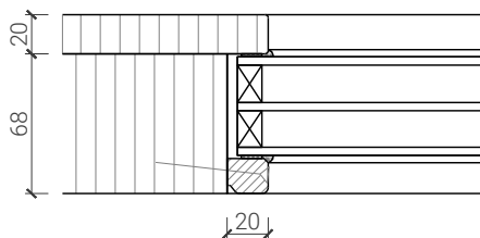
Glas mittig, 68 mm Glasleiste einseitig
