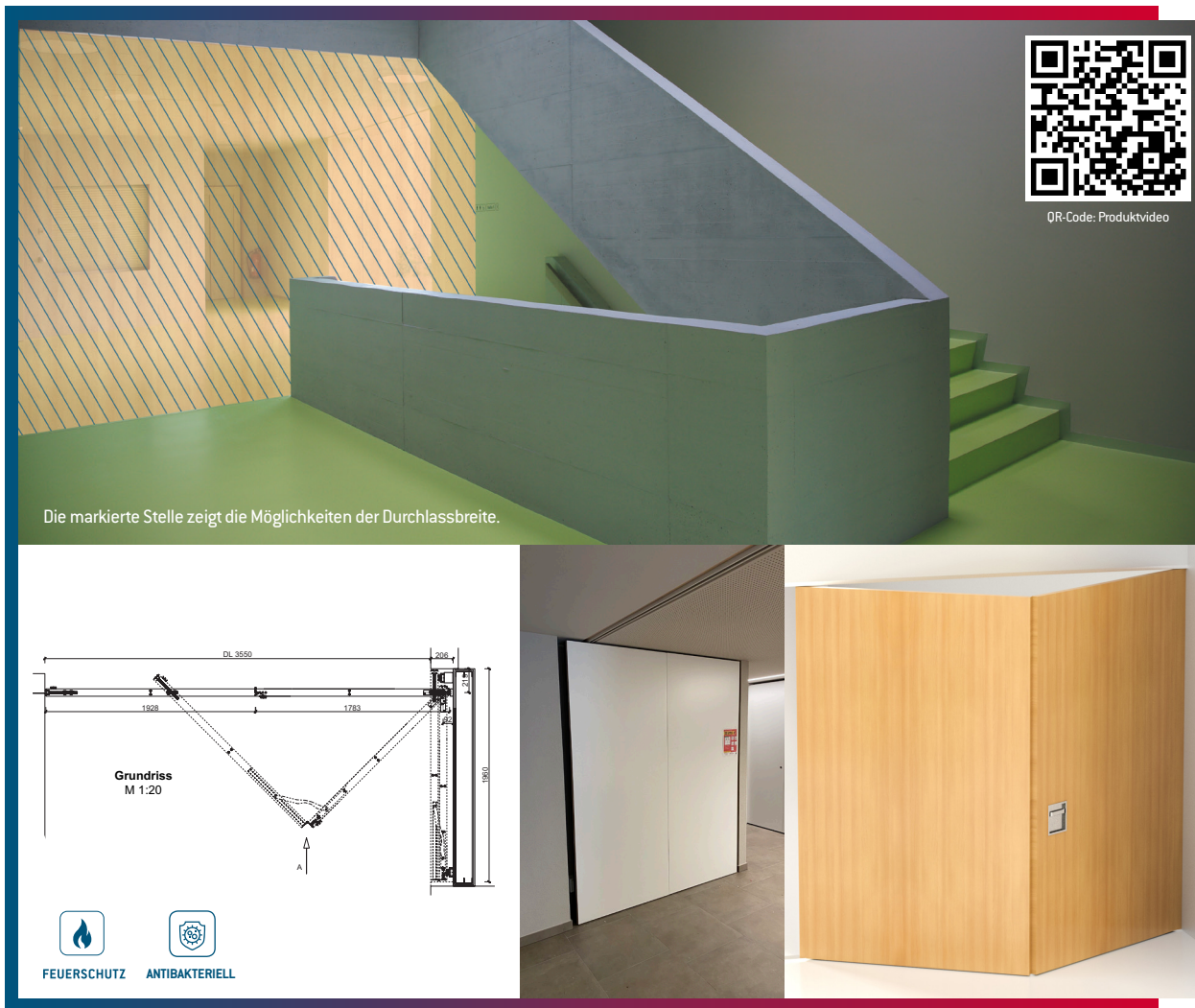
STURM FALT-SCHIEBETÜR (EI30) Brandschutz wurde speziell zum Abschotten oder Verschließen großer Wandöffnungen entwickelt.
