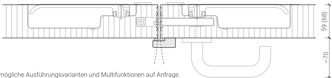
Variante Mittelschlag - Pendeltür mit Panikschloss
