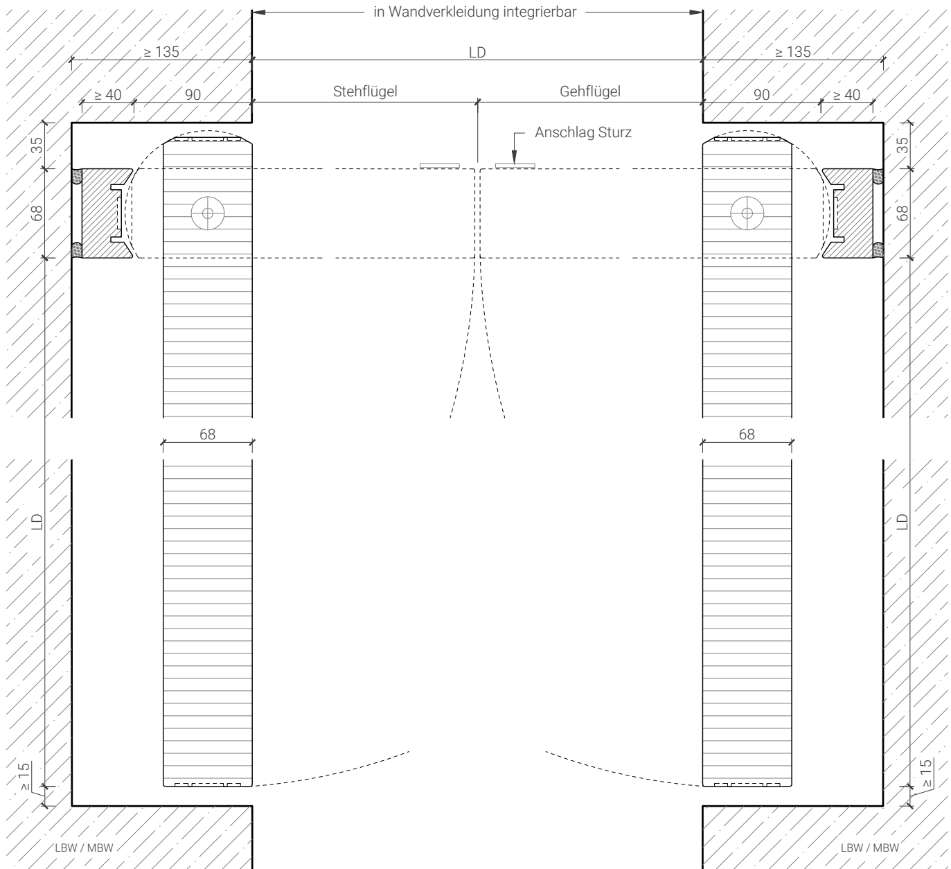
Variante Mittelschlag - Pendeltür 68 mm mit Panikschloss
