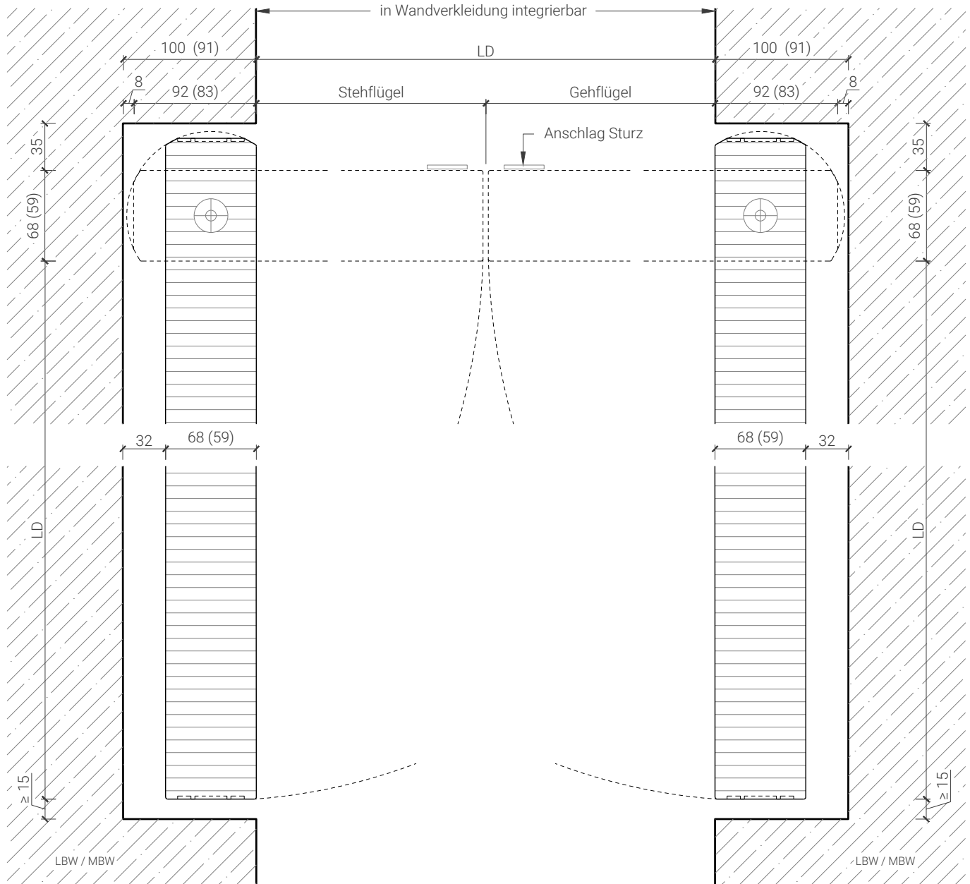
Variante Mittelschlag - Pendeltür mit Panikschloss
