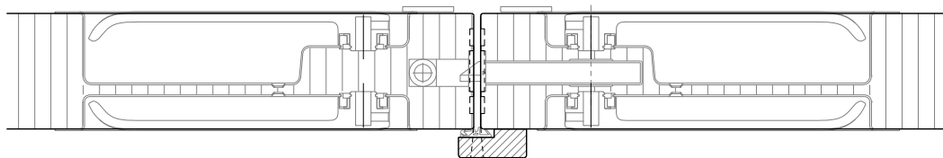
Variante Mittelschlag - Pendeltür 68 mm mit Panikschloss
