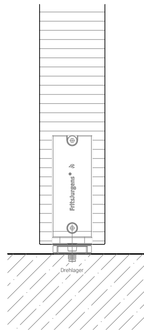
Bodendrehlager mit int. Türschließer FritsJürgens
