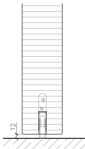
Streiftüre mit Bodendichtung
