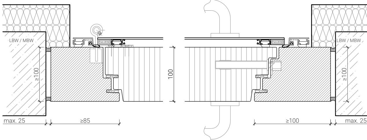
Blockrahmen 100 mm mit Blindstock, Türe stumpf nach aussen öffnend
