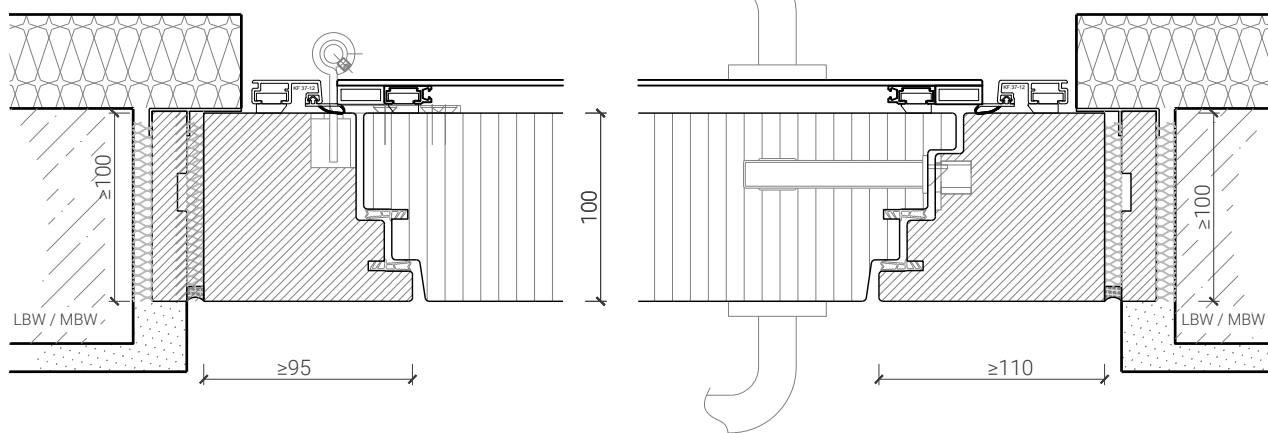
Blockrahmen 100 mm mit Blindstock, Türe stumpf nach aussen öffnend
