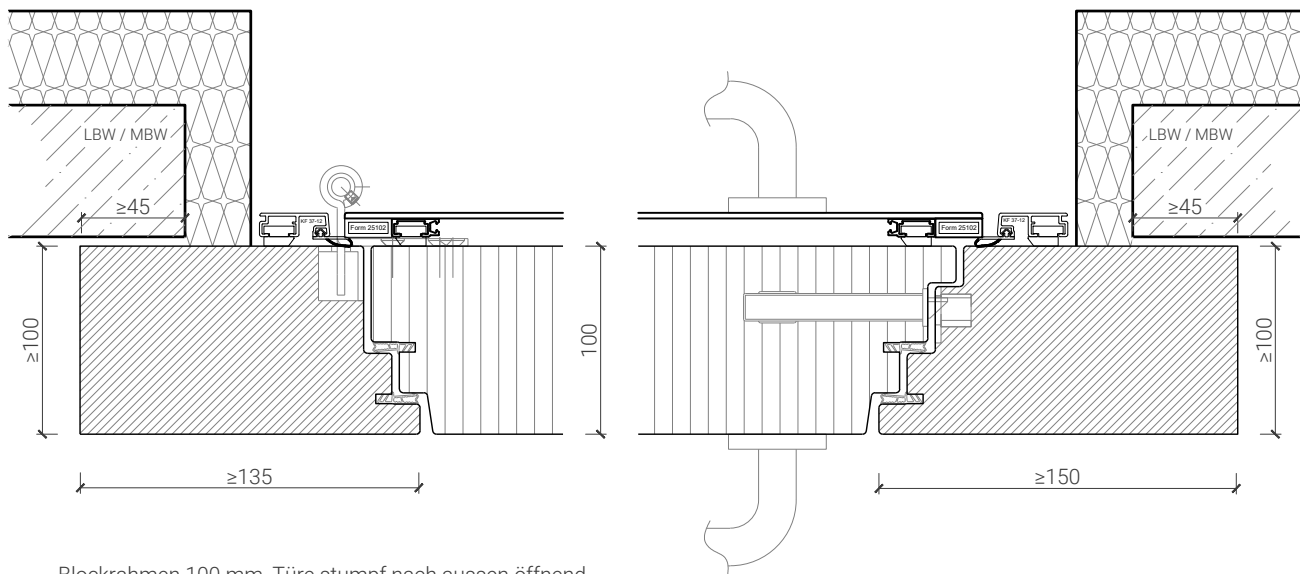
Blockrahmen 100 mm, Türe stumpf nach aussen öffnend
