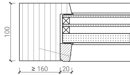
Glaslichtkante Sperrholz/HDF Glasleiste einseitig
