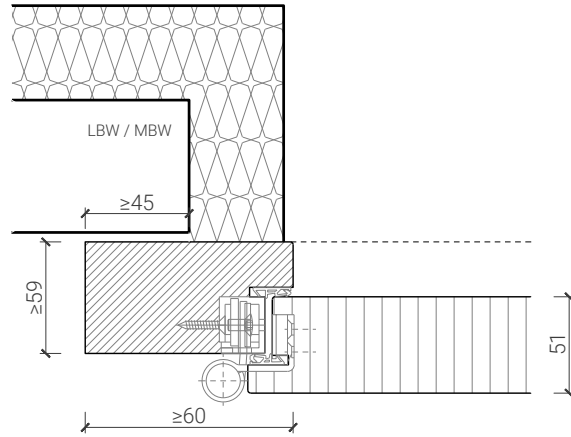
Blendrahmen 68 mm, Türe gefälzt
