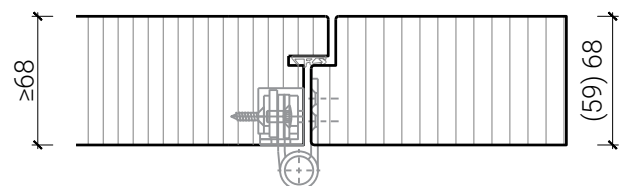
Einbau in Vollwand, Türe stumpf
