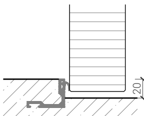
Anschlagwinkel mit Dichtung 40x30*
