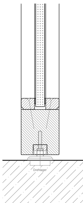
Bodendrehlager
