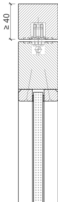
Bodentürschließer
