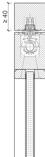
Bodendrehlager
