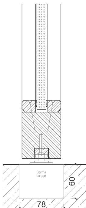
Bodentürschließer
