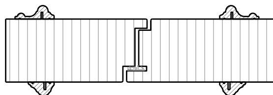
EI60 / EI90 Mittelanschlag, Schlagleisten profiliert
