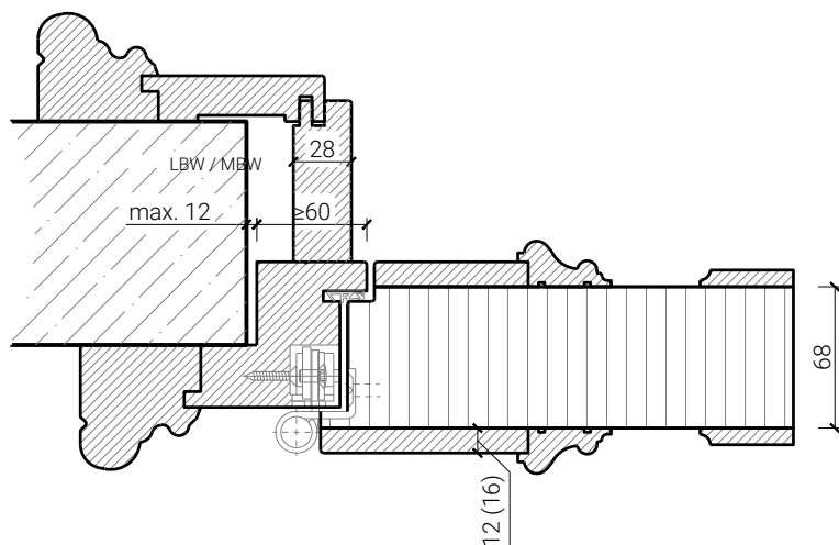
EI60 - Blockrahmen mit Umfassungsfutter, Türe gefälzt
