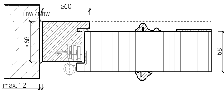
EI60 - Blockrahmen mit Umfassungsfutter, Türe gefälzt
