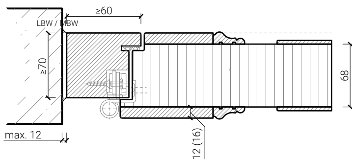
EI60 / EI90 - Blockrahmen, Türe gefälzt
