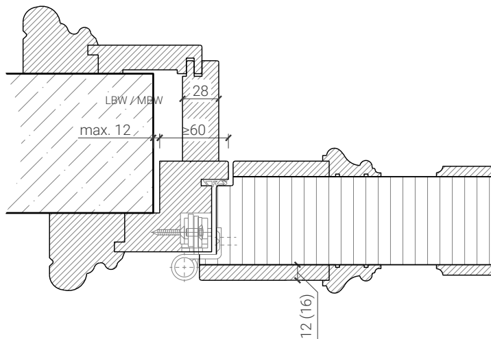
EI60 - Blockrahmen mit Umfassungsfutter, Türe gefälzt
